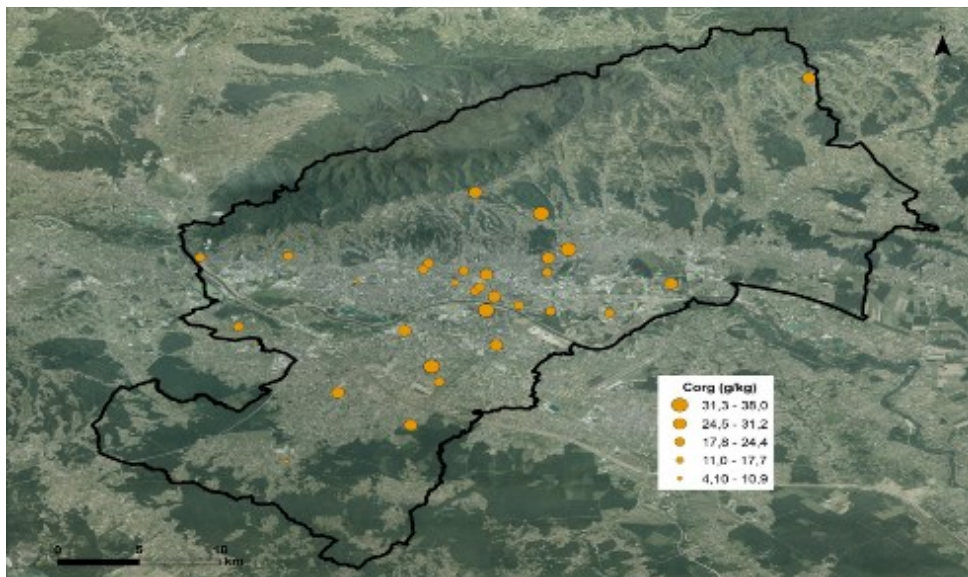
Slika 4 – Raspodjela vrijednosti organskog ugljika ( C_{\text{org}} ) u urbanom tlu uzorkovanom 2025. g.
