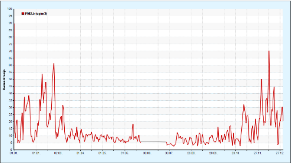
Slika 7 – Grafički prikaz kretanja 24-satnih koncentracija PM_{2,5} frakcije lebdećih čestica na mjernoj postaji Mirogojska cesta tijekom 2025. godine
