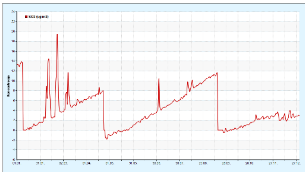
Slika 2 – Grafički prikaz 24-satnih koncentracija sumporovog dioksida \text{SO}_2 na mjernoj postaji Mirogojska cesta
